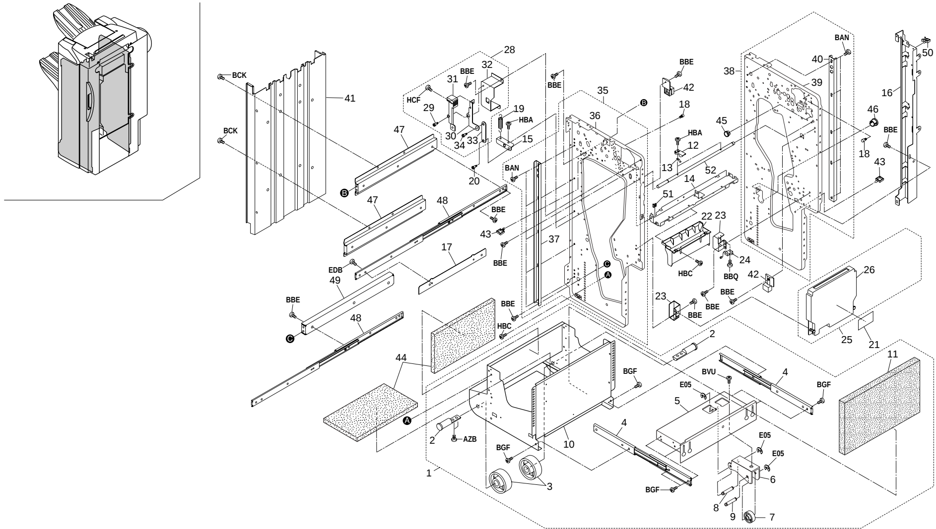
FIG. 2 FRAMES
