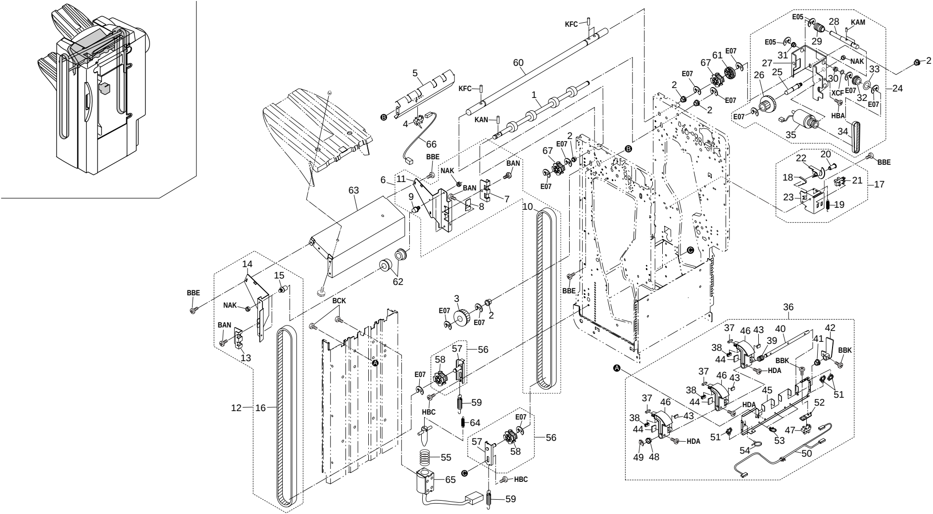
FIG. 3 BIN SECTION
